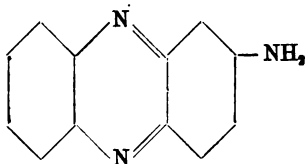
Aminophenazin.
